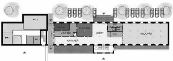
Pôdorys 1. NP
